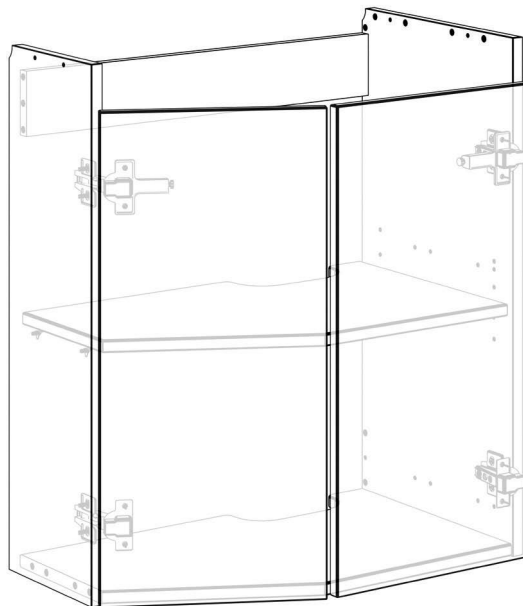
Allaskaappi | Tvättställsskåp | Washbasin Cabinet
